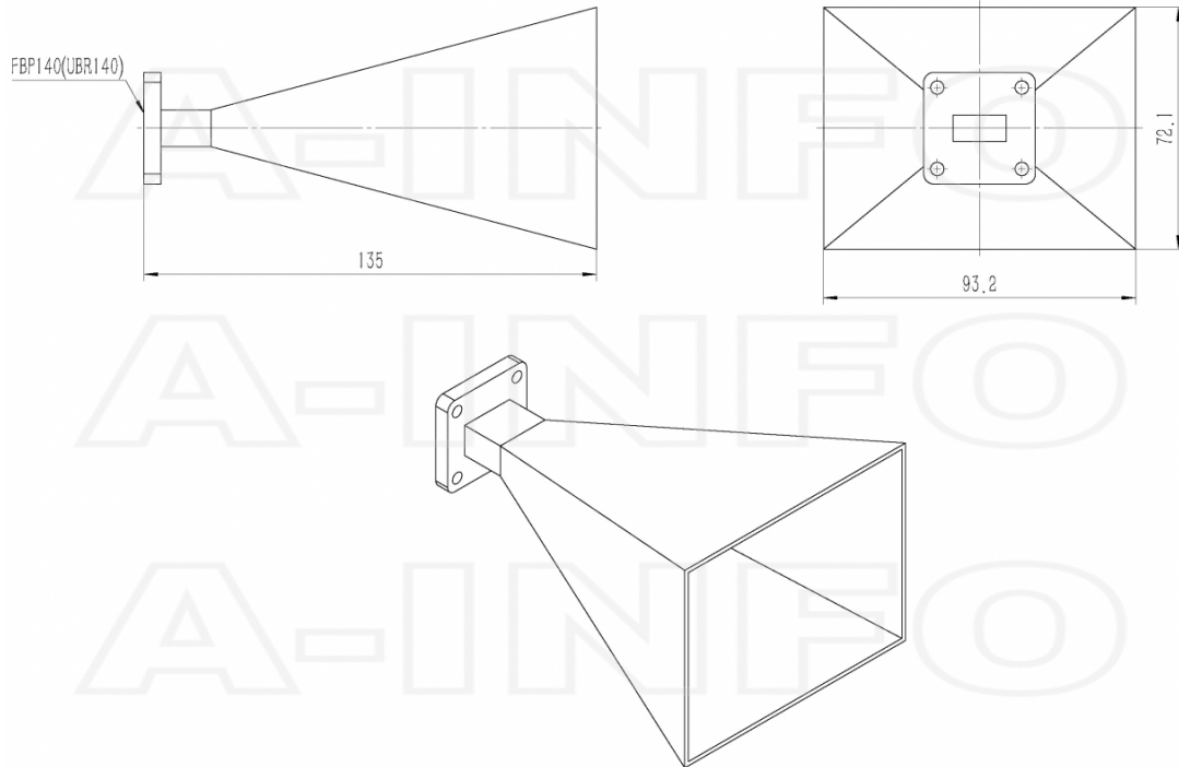
FBP140 Output (P/N: LB-62-20-A)
